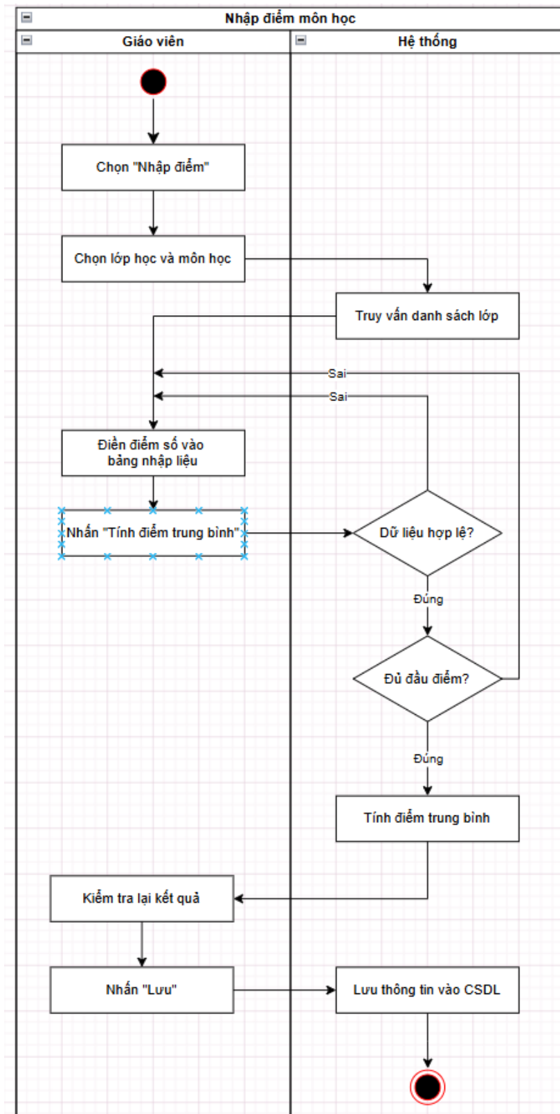
Biểu đồ hoạt động: nhập điểm môn học
