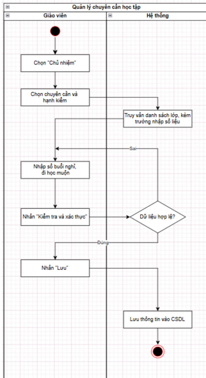
Biểu đồ hoạt động: quản lý chuyên cần học tập
