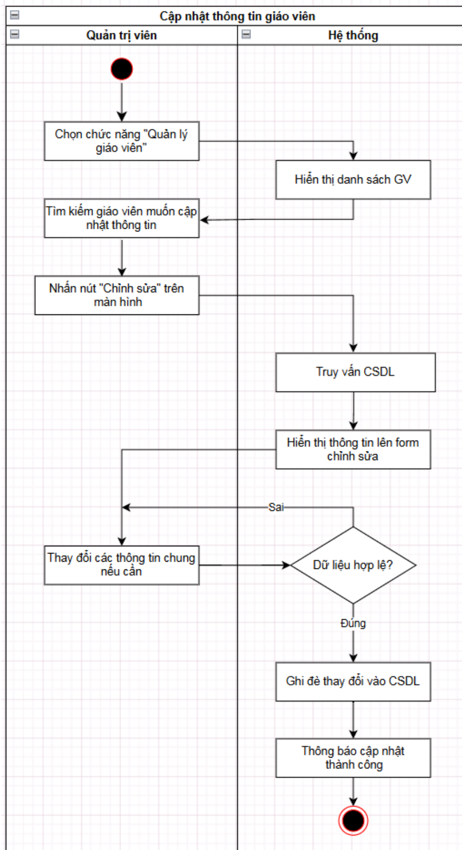
Biểu đồ hoạt động: Cập nhật thông tin giáo viên
