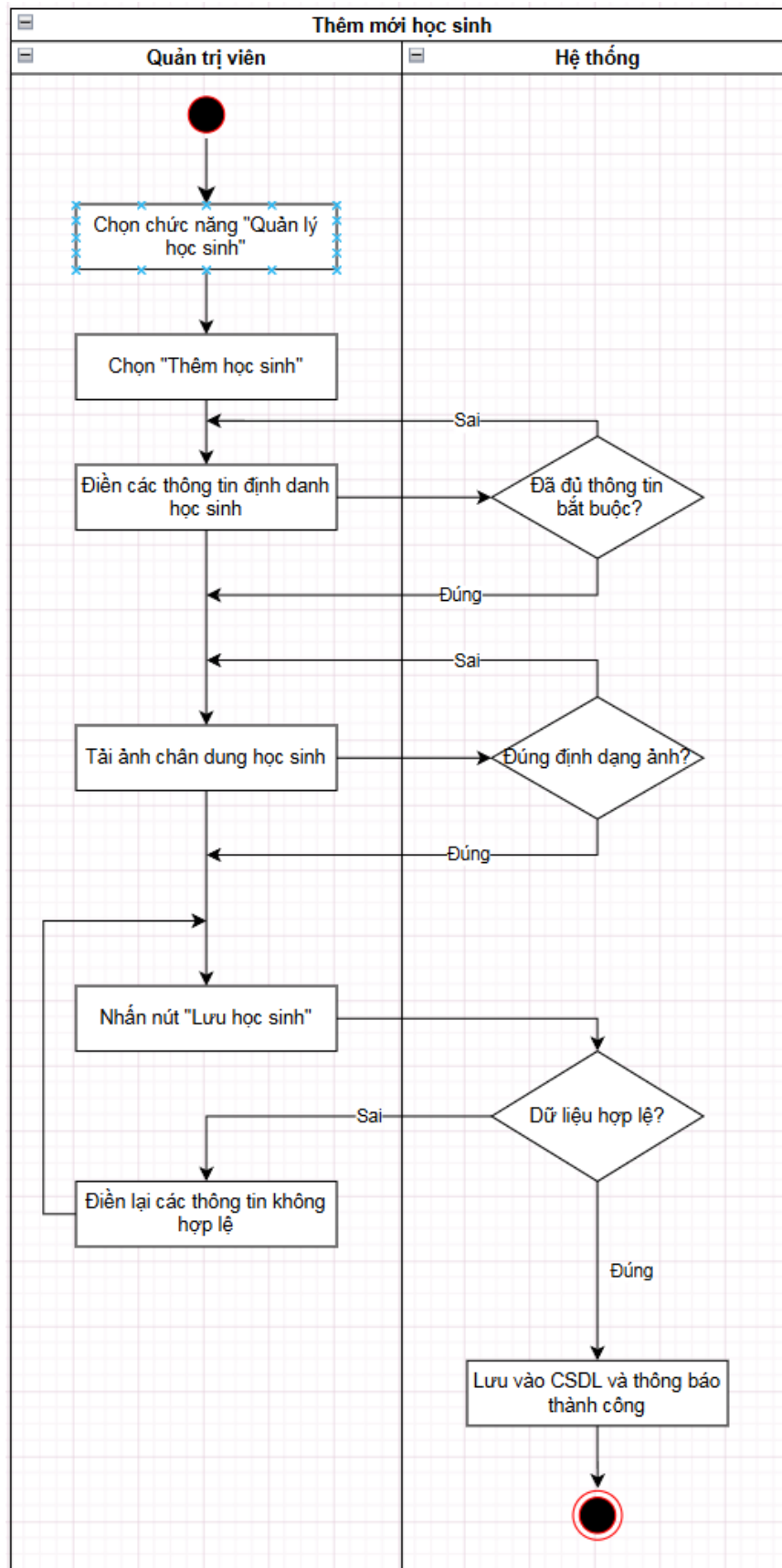
Biểu đồ hoạt động: Quy trình thêm mới học sinh
