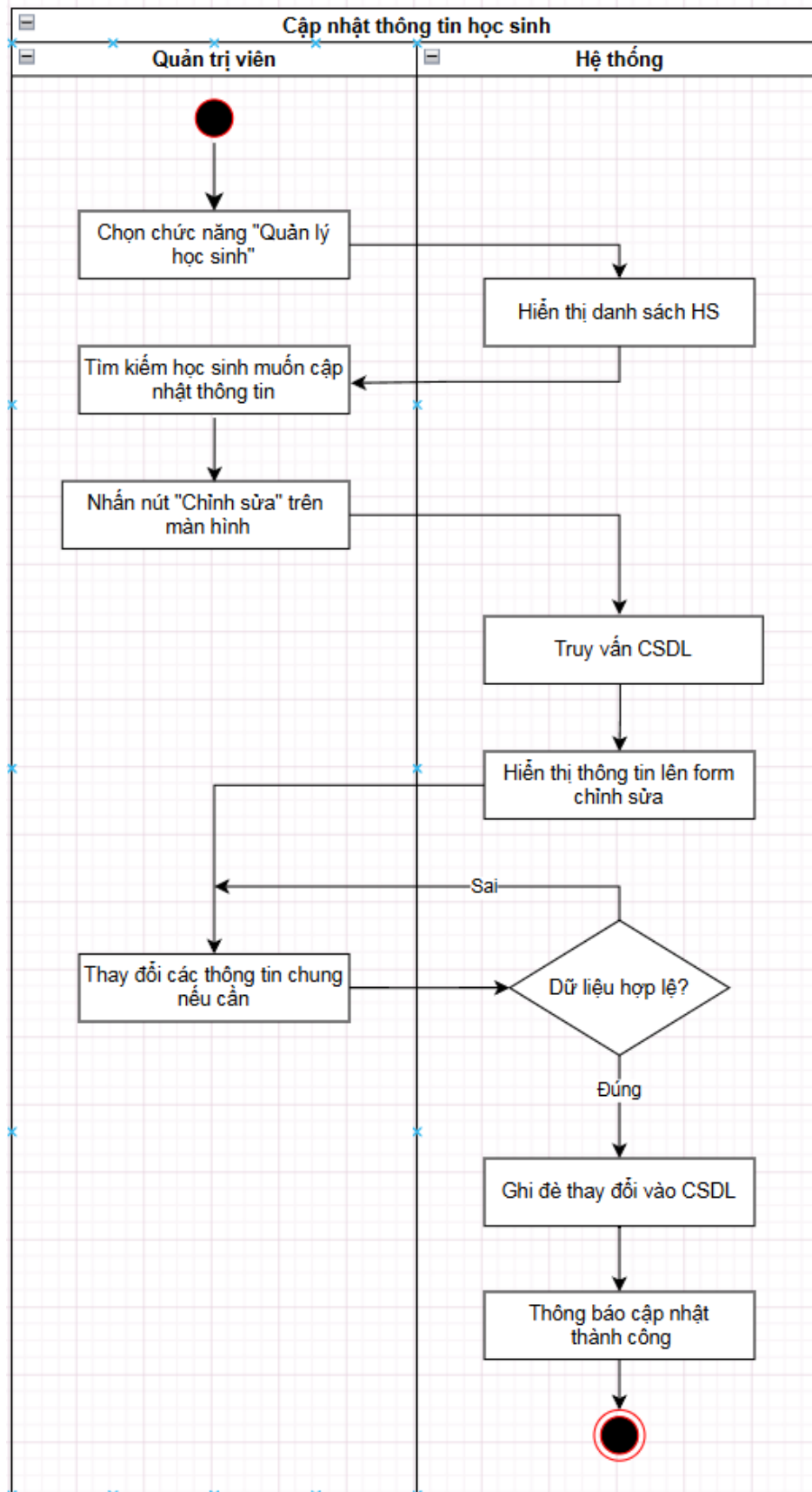
Biểu đồ hoạt động: Cập nhật thông tin học sinh
