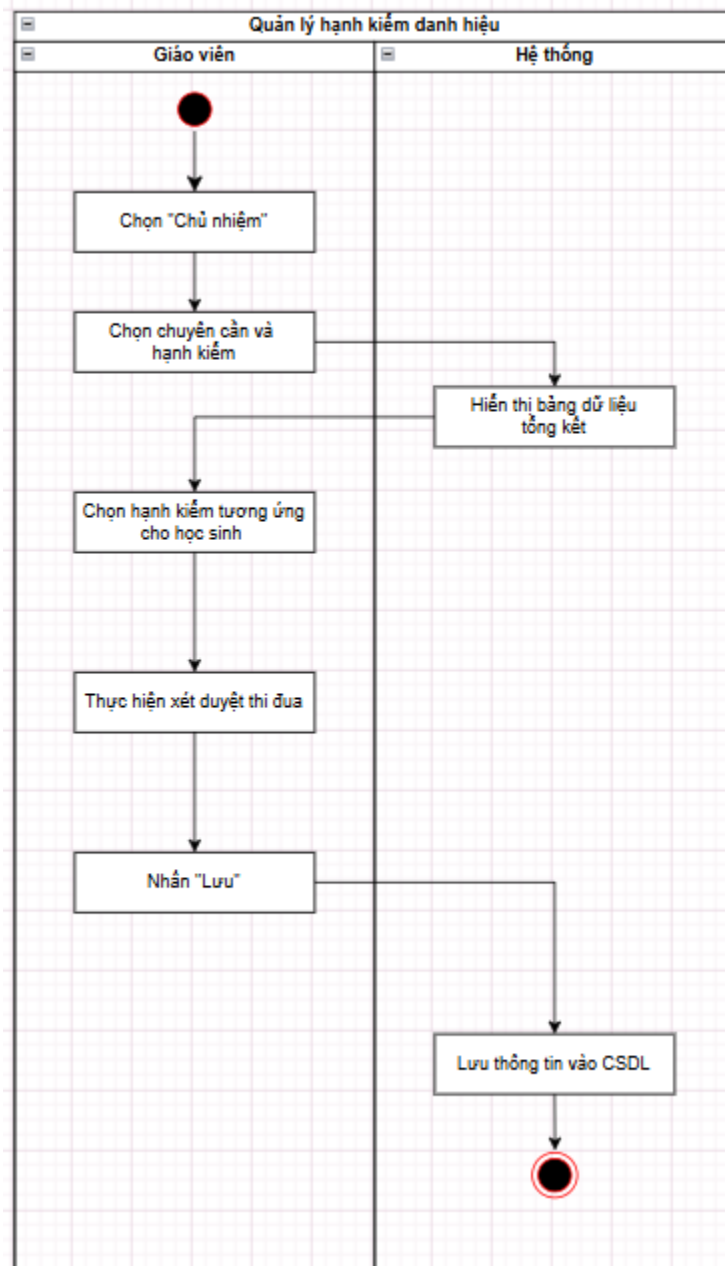
Biểu đồ hoạt động: quản lý hạnh kiểm và danh hiệu
